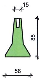
Schnitt
